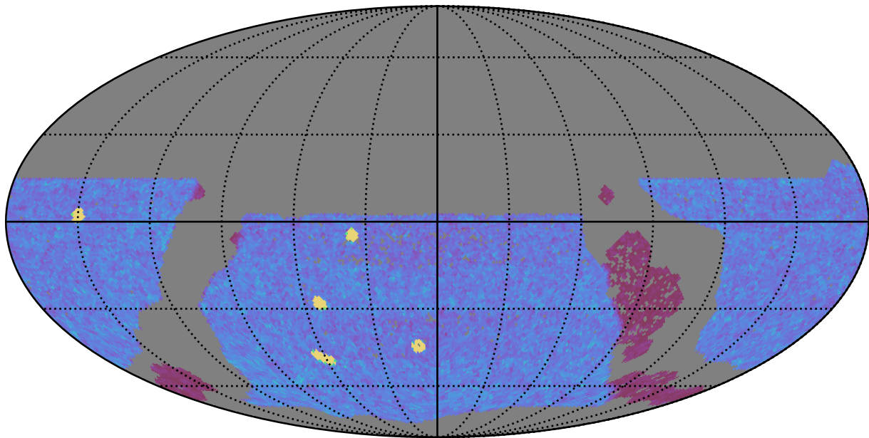
too_elab_r8_d3_ugrizy_v3.4_10yrs WFD y band: NVisits
