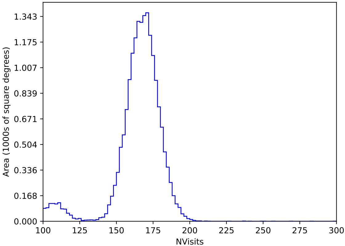
too_elab_r8_d3_ugrizy_v3.4_10yrs WFD y band: NVisits
