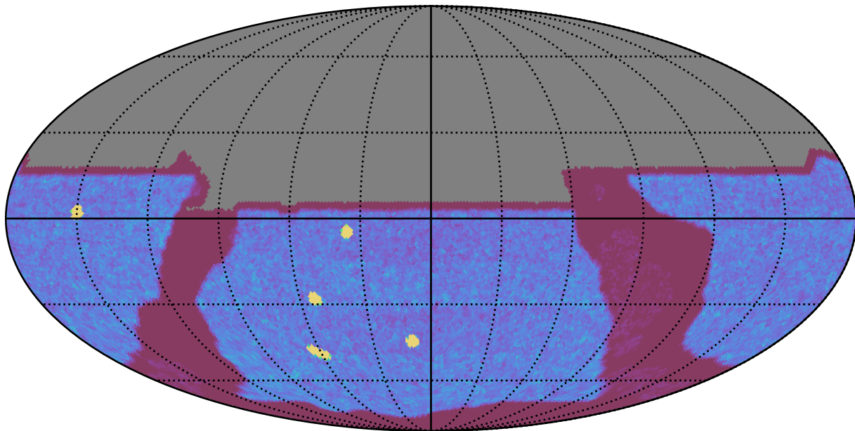
too_elab_r8_d3_ugrizy_v3.4_10yrs All sky y band: NVisits
