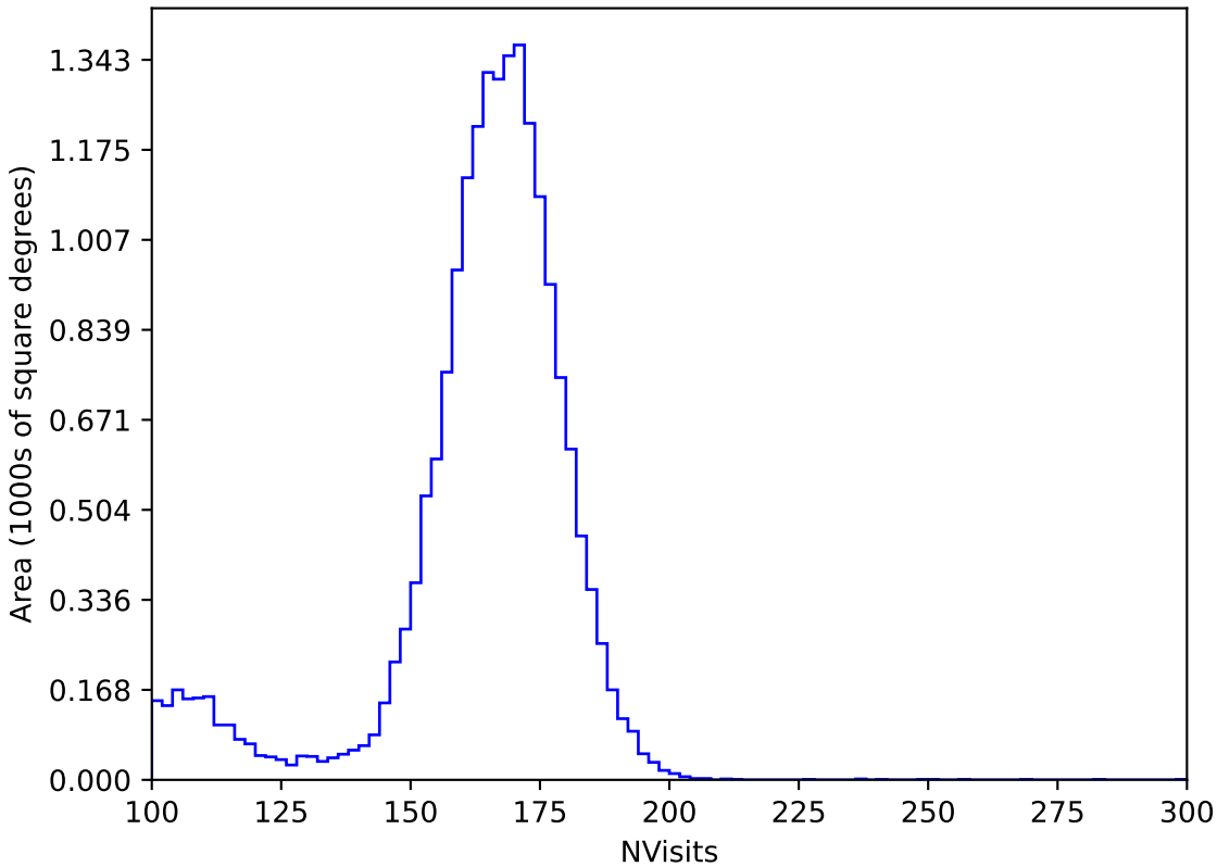
too_elab_r8_d3_ugrizy_v3.4_10yrs All sky y band: NVisits
