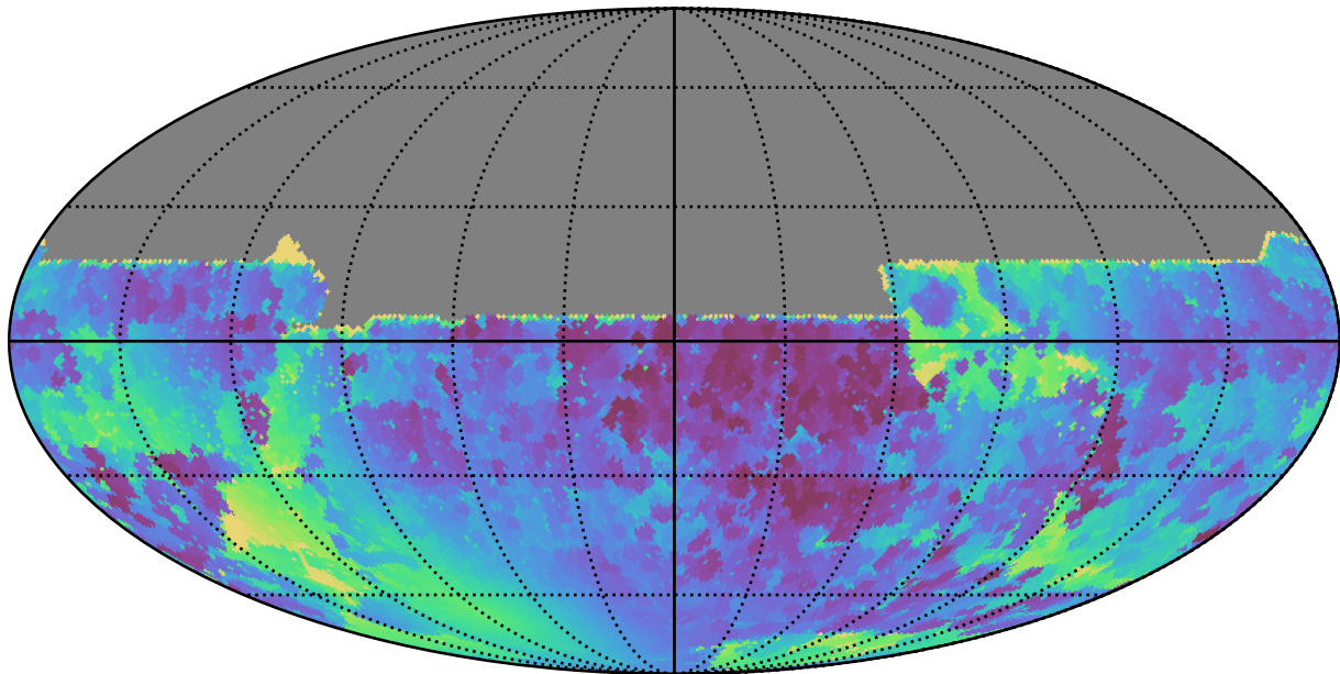
too_elab_r8_d3_ugrizy_v3.4_10yrs All sky y band: Min solarElong
