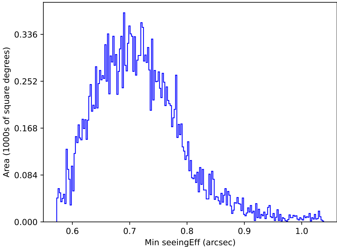
too_elab_r8_d3_ugrizy_v3.4_10yrs Yr 1 y band: Min seeingEff
