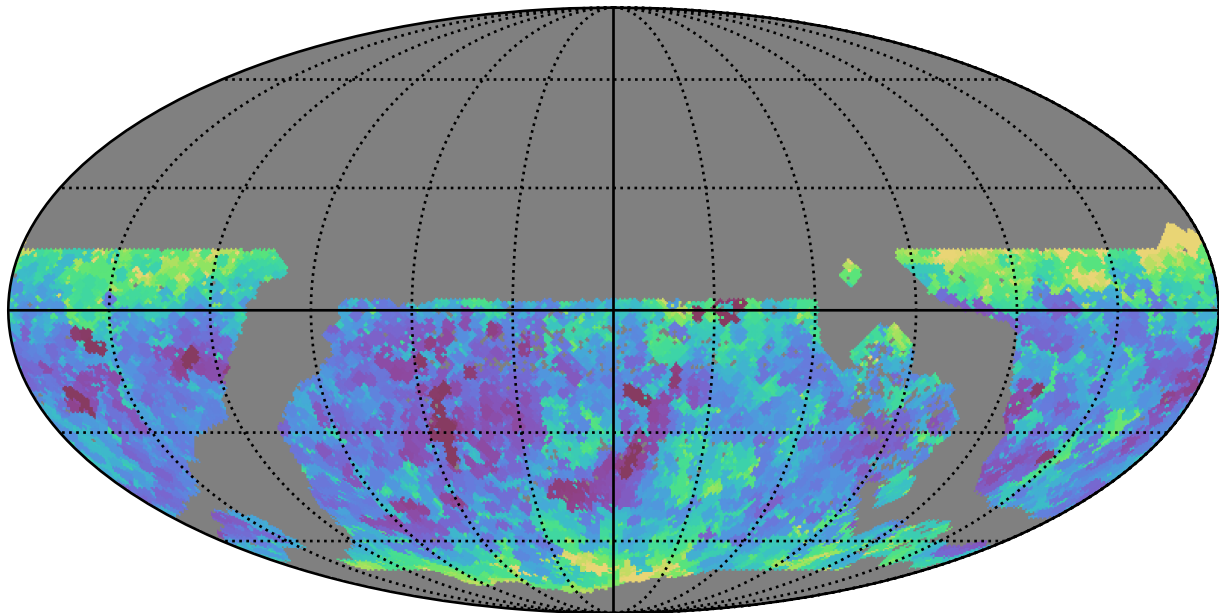
too_elab_r8_d3_ugrizy_v3.4_10yrs WFD y band: Min seeingEff
