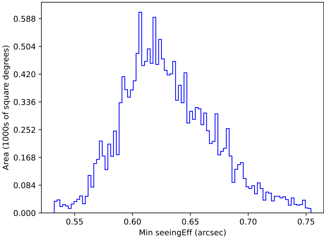
too_elab_r8_d3_ugrizy_v3.4_10yrs WFD y band: Min seeingEff
