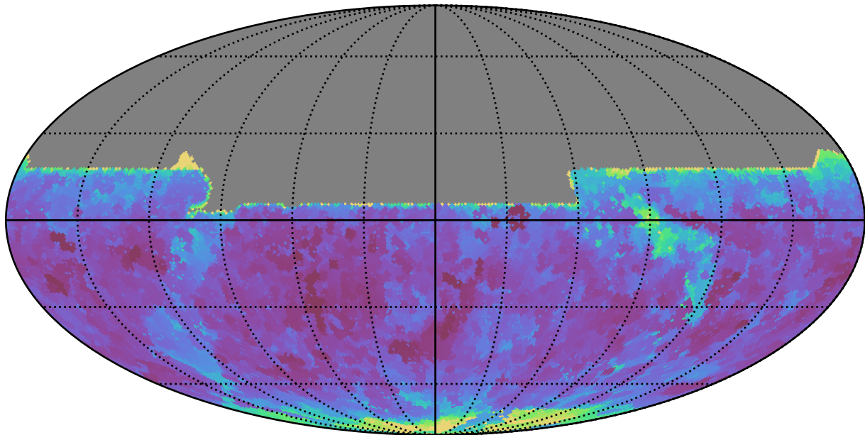
too_elab_r8_d3_ugrizy_v3.4_10yrs All sky y band: Min seeingEff
