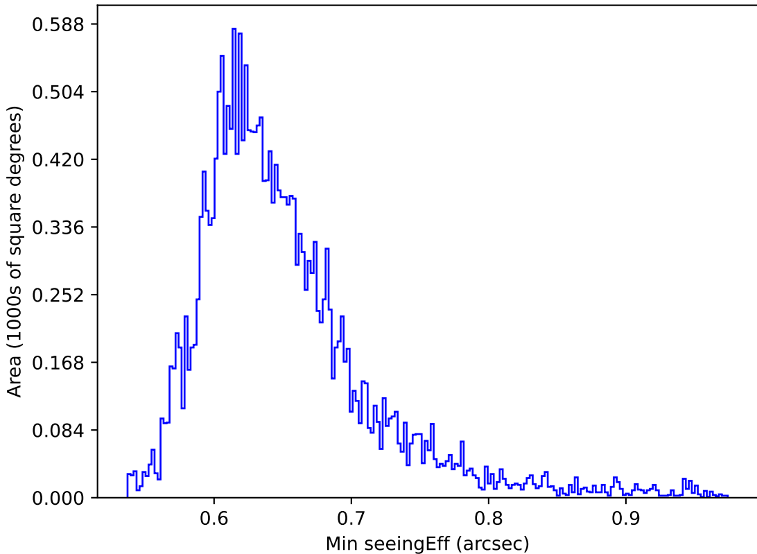
too_elab_r8_d3_ugrizy_v3.4_10yrs All sky y band: Min seeingEff
