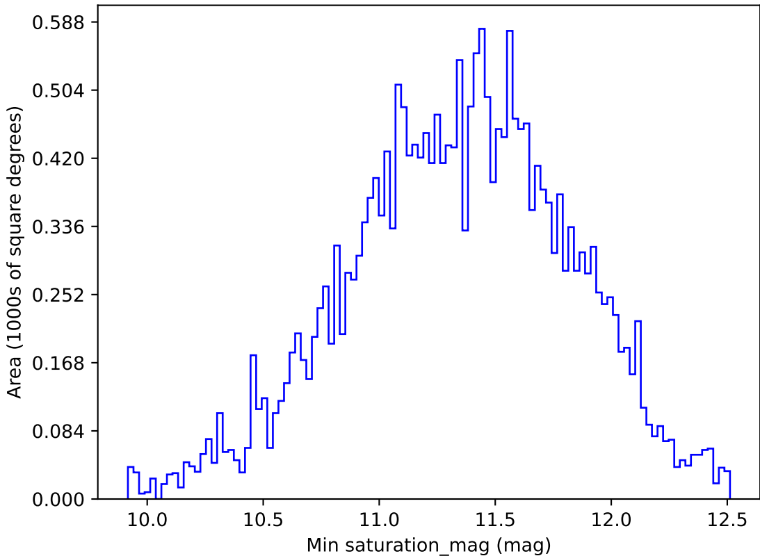
too_elab_r8_d3_ugrizy_v3.4_10yrs All sky y band: Min saturation_mag
