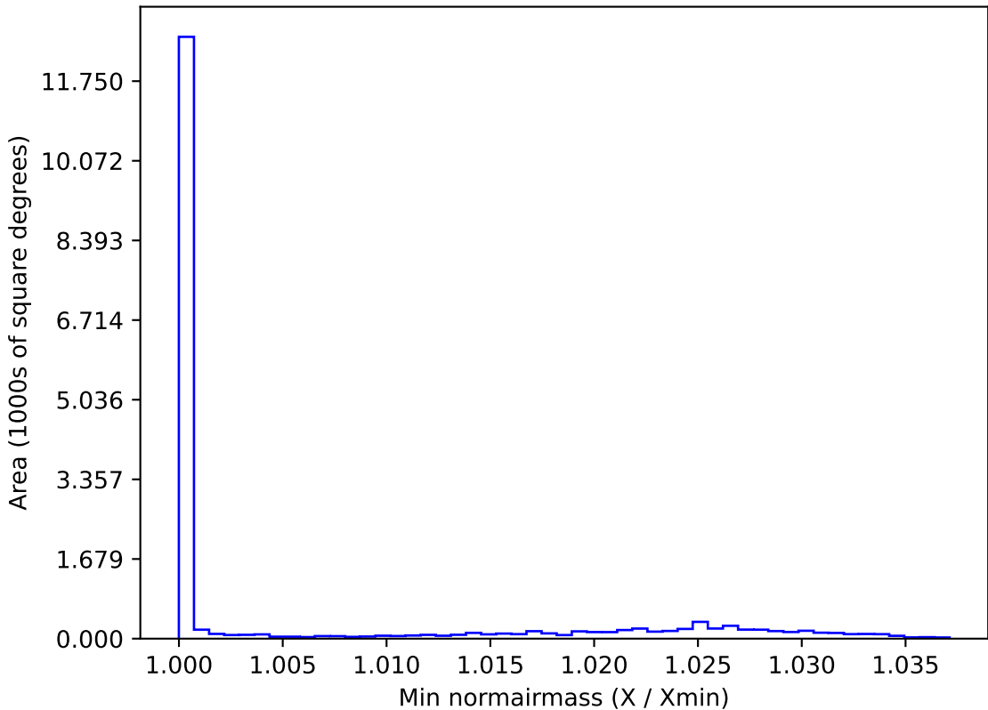
too_elab_r8_d3_ugrizy_v3.4_10yrs WFD z band: Min normairmass
