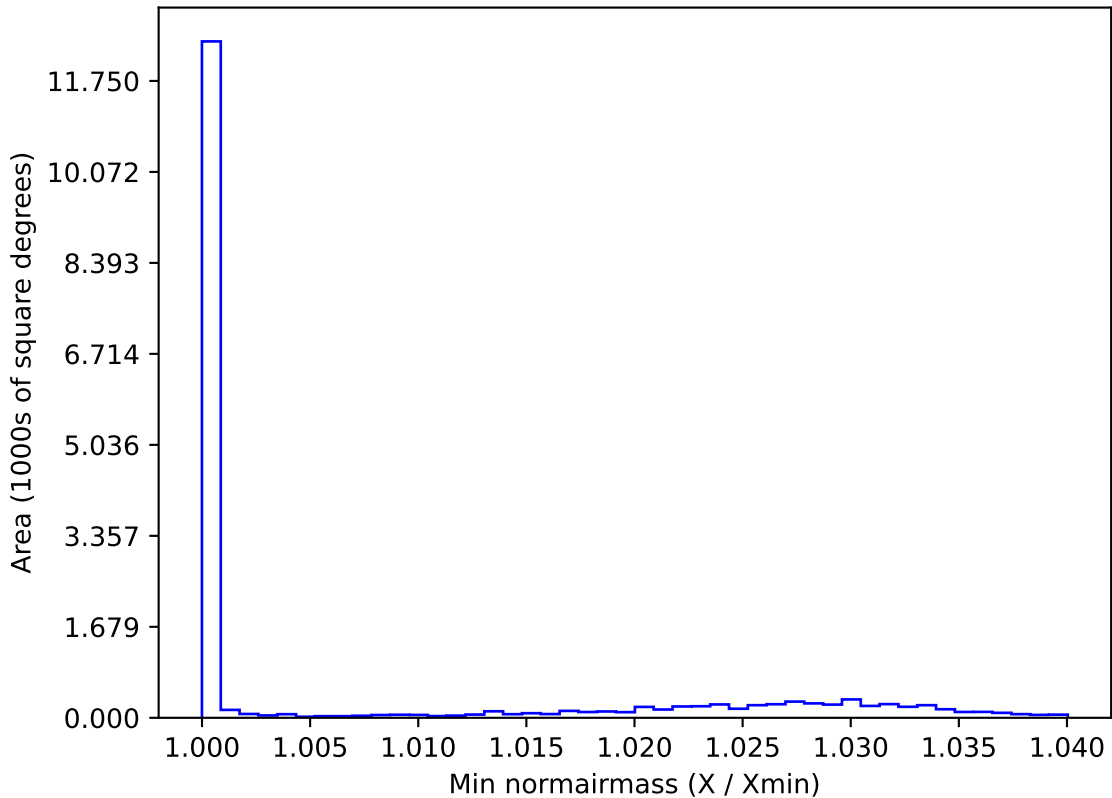
too_elab_r8_d3_ugrizy_v3.4_10yrs WFD y band: Min normairmass
