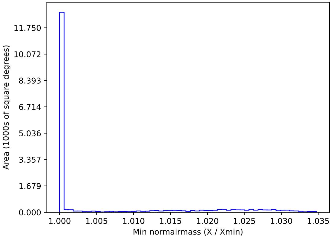
too_elab_r8_d3_ugrizy_v3.4_10yrs WFD r band: Min normairmass
