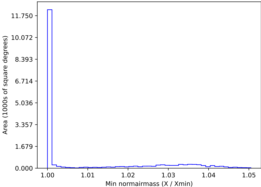
too_elab_r8_d3_ugrizy_v3.4_10yrs WFD g band: Min normairmass
