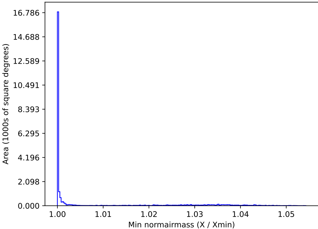
too_elab_r8_d3_ugrizy_v3.4_10yrs All sky g band: Min normairmass
