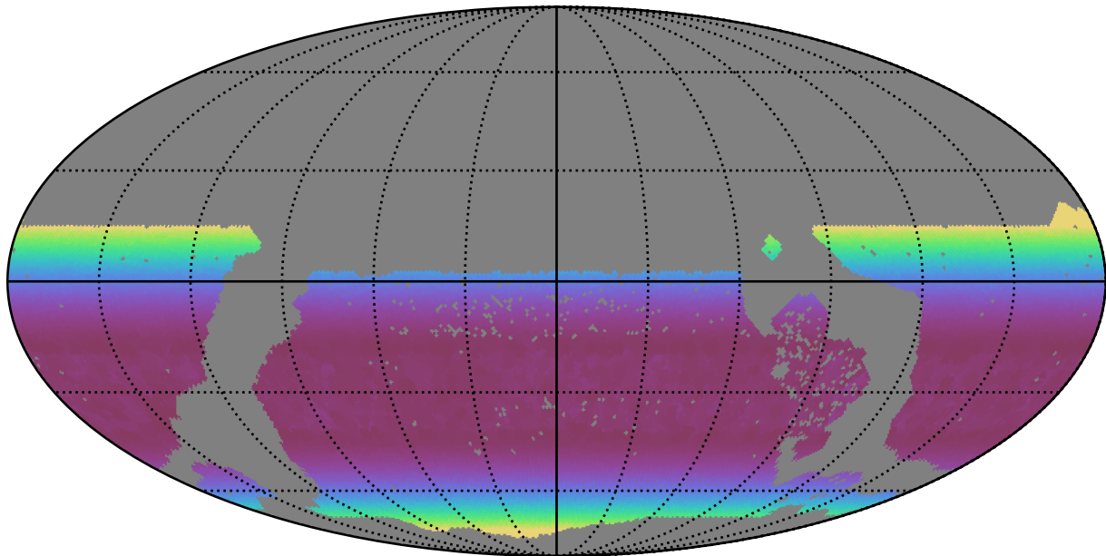
too_elab_r8_d3_ugrizy_v3.4_10yrs WFD y band: Min airmass
