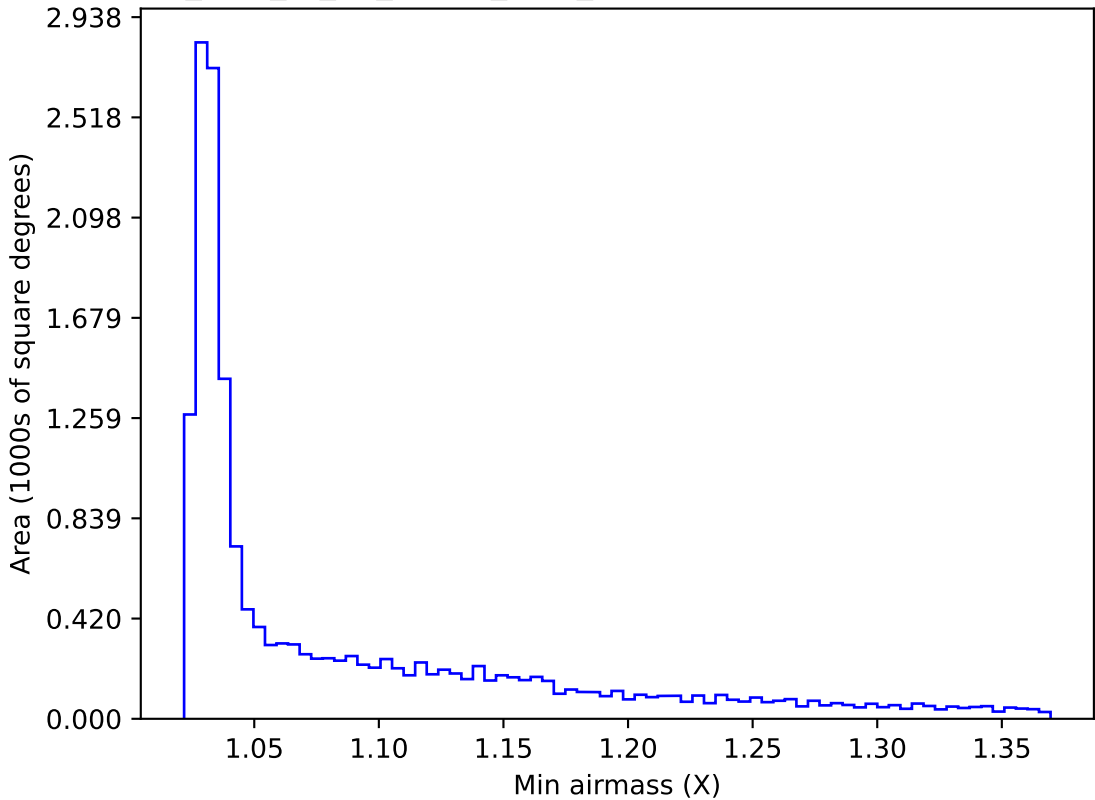
too_elab_r8_d3_uigrzy_v3.4_10yrs WFD y band: Min airmass
