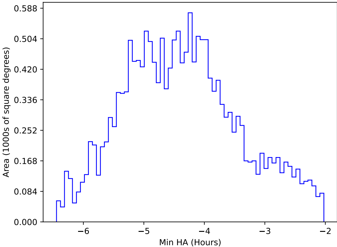
too_elab_r8_d3_ugrizy_v3.4_10yrs WFD z band: Min HA
