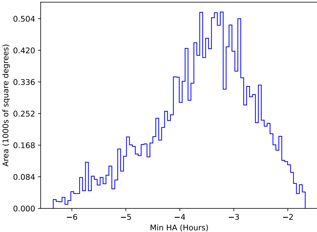
too_elab_r8_d3_ugrizy_v3.4_10yrs WFD y band: Min HA
