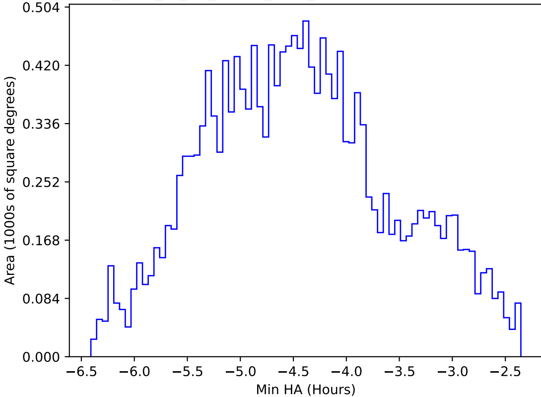
too_elab_r8_d3_ugrizy_v3.4_10yrs WFD r band: Min HA
