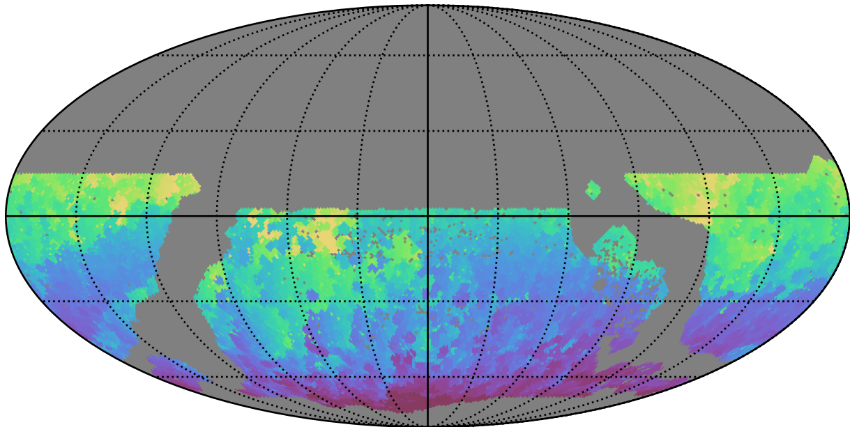
too_elab_r8_d3_ugrizy_v3.4_10yrs WFD i band: Min HA
