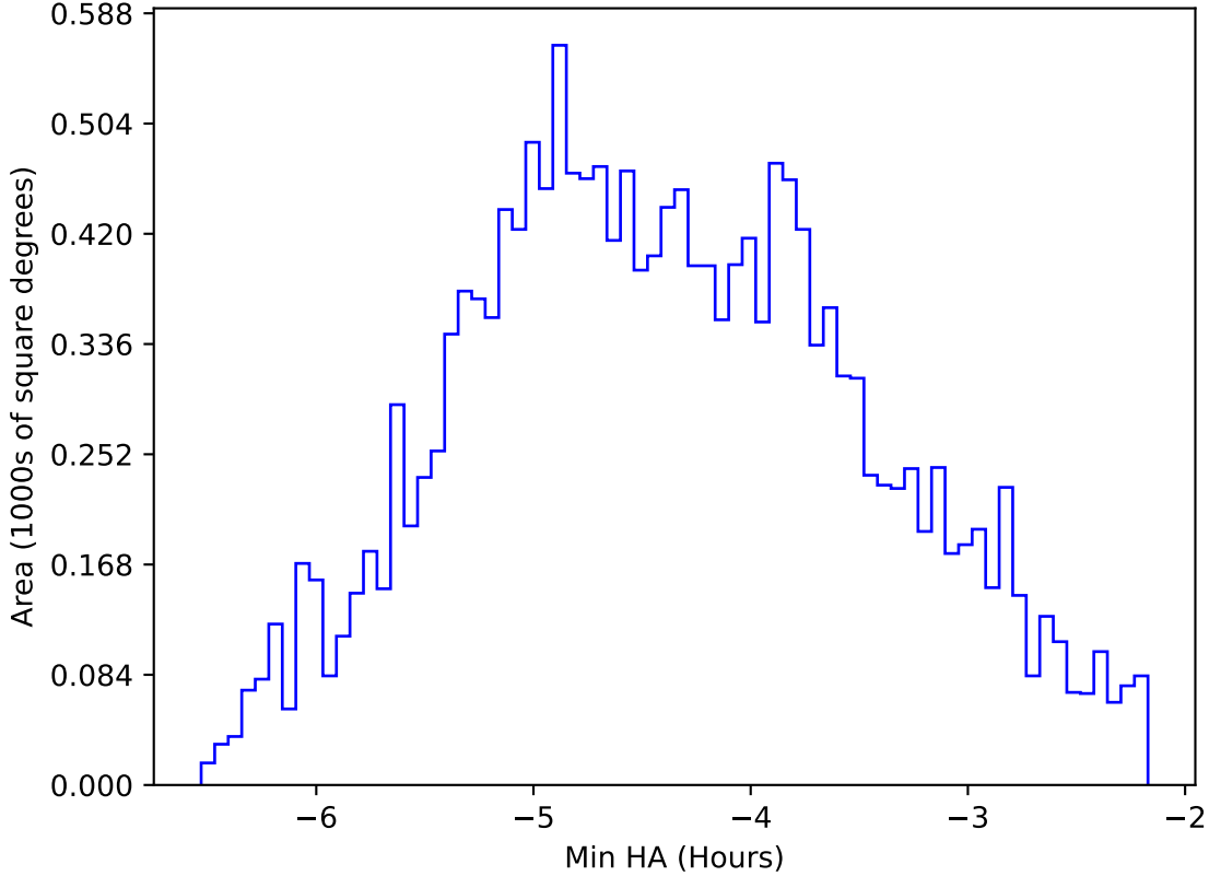
too_elab_r8_d3_ugrizy_v3.4_10yrs WFD i band: Min HA
