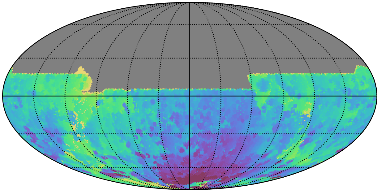
too_elab_r8_d3_ugrizy_v3.4_10yrs All sky y band: Min HA
