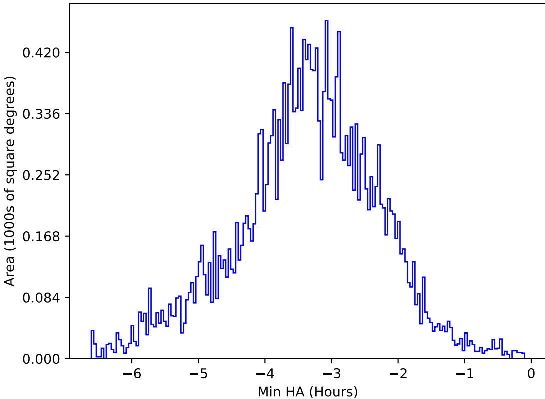
too_elab_r8_d3_ugrizy_v3.4_10yrs All sky y band: Min HA
