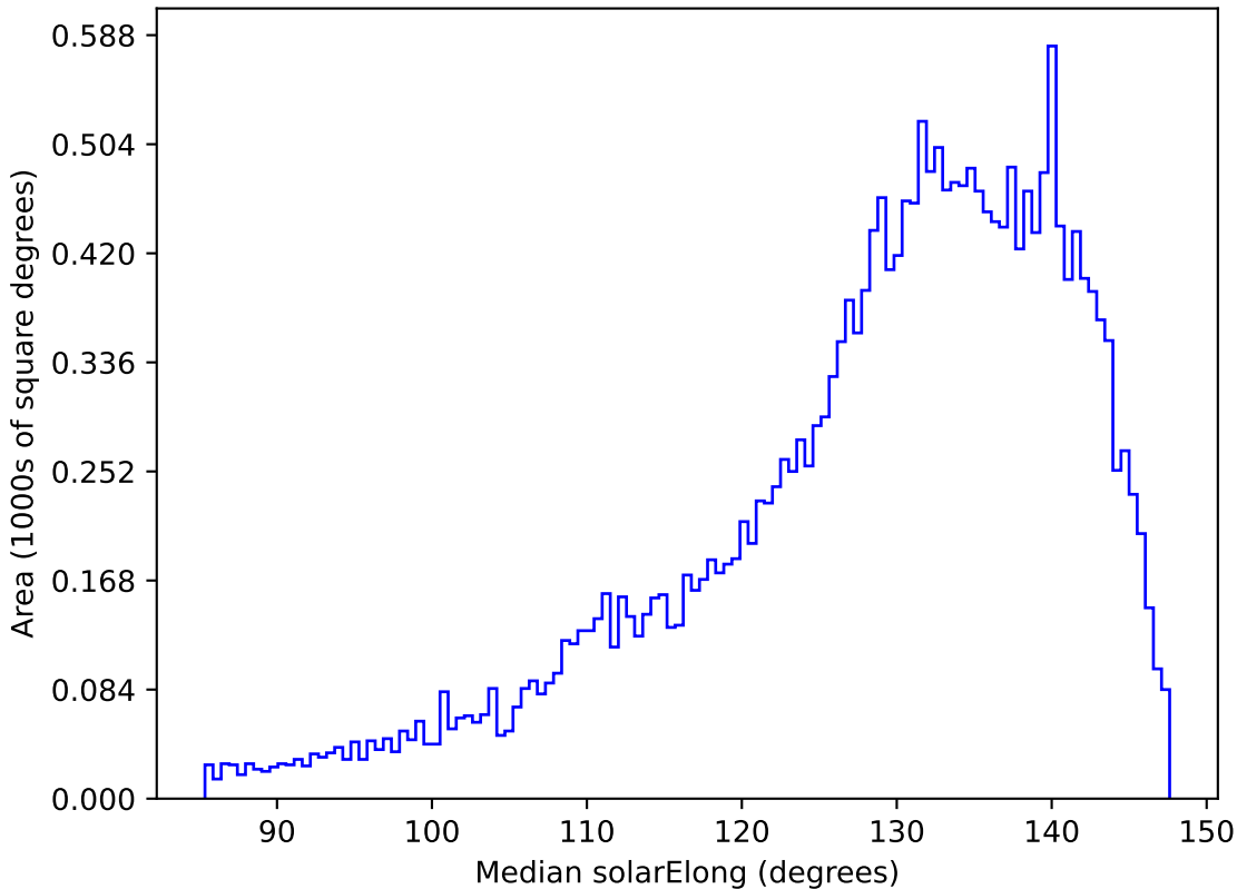
too_elab_r8_d3_ugrizy_v3.4_10yrs All sky y band: Median solarElong
