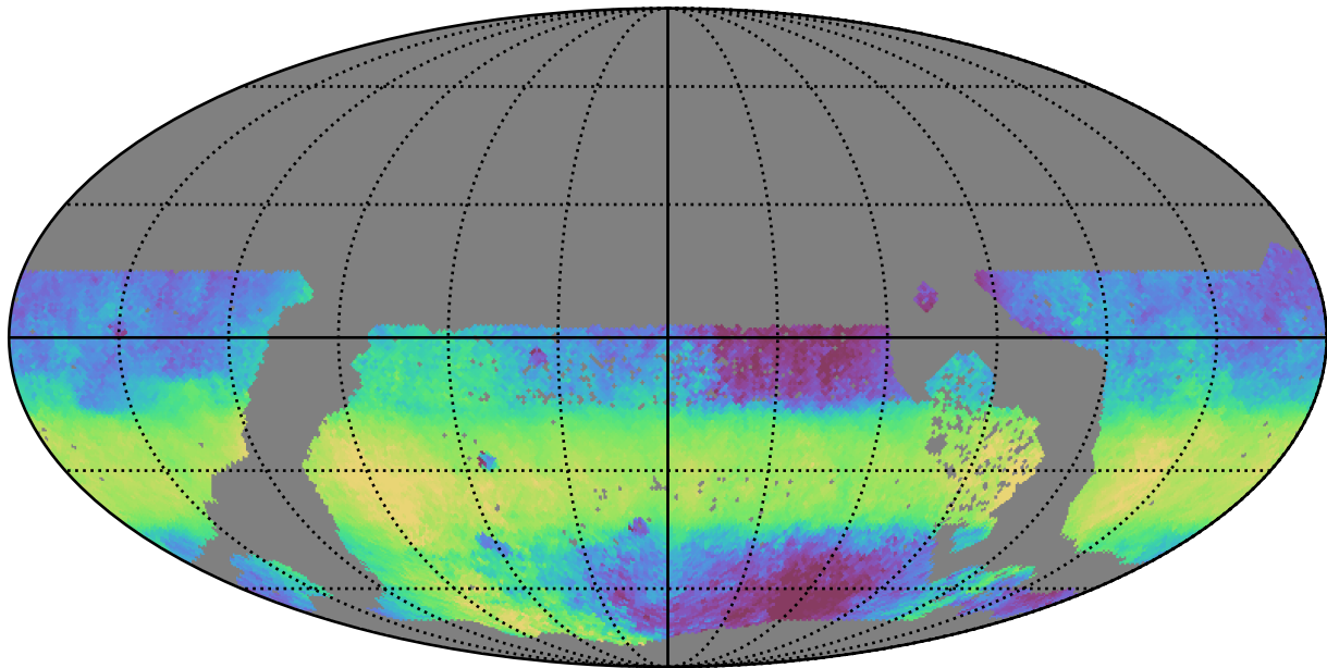
too_elab_r8_d3_ugrizy_v3.4_10yrs WFD y band: Median HA
