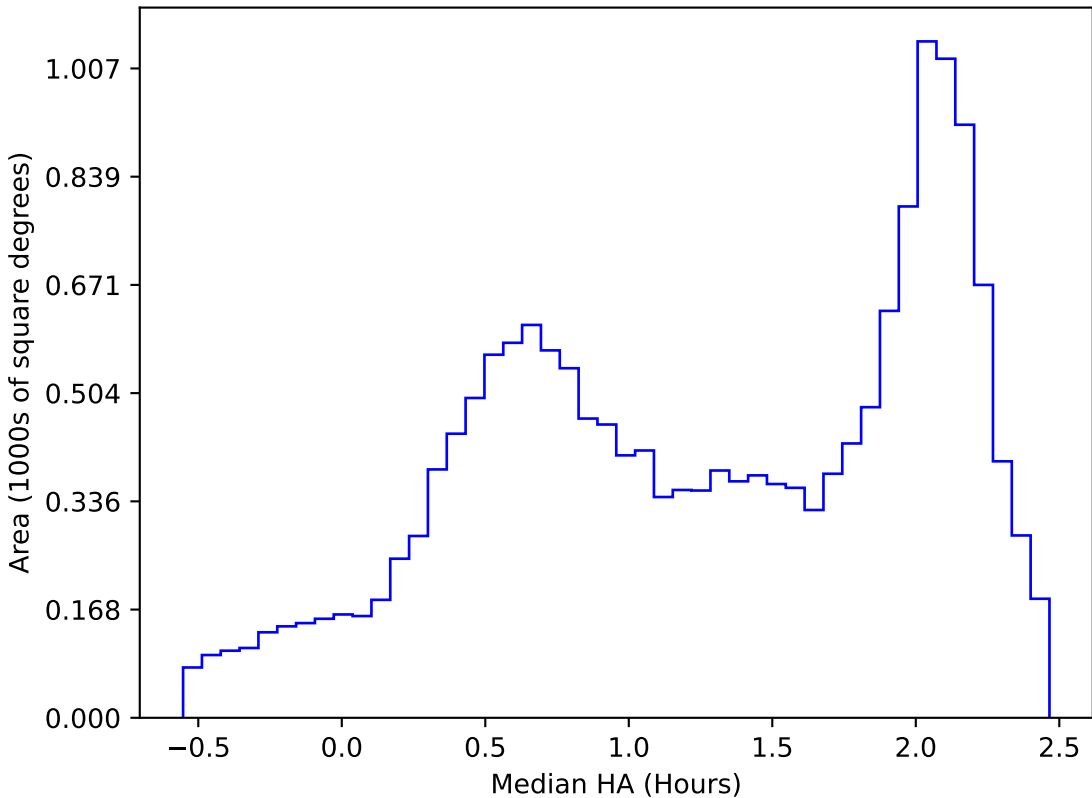
too_elab_r8_d3_ugrizy_v3.4_10yrs WFD y band: Median HA
