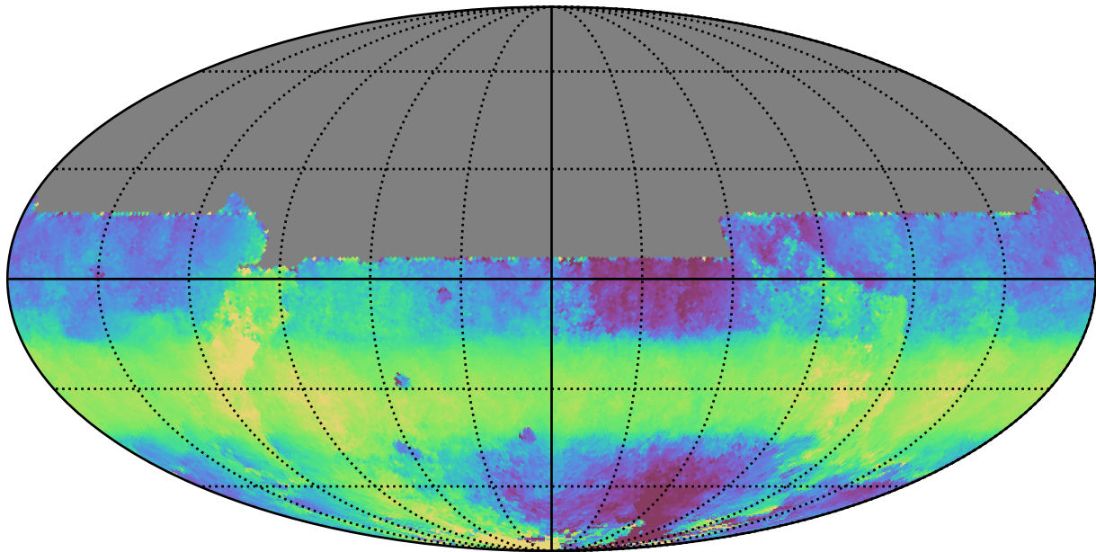
too_elab_r8_d3_ugrizy_v3.4_10yrs All sky y band: Median HA
