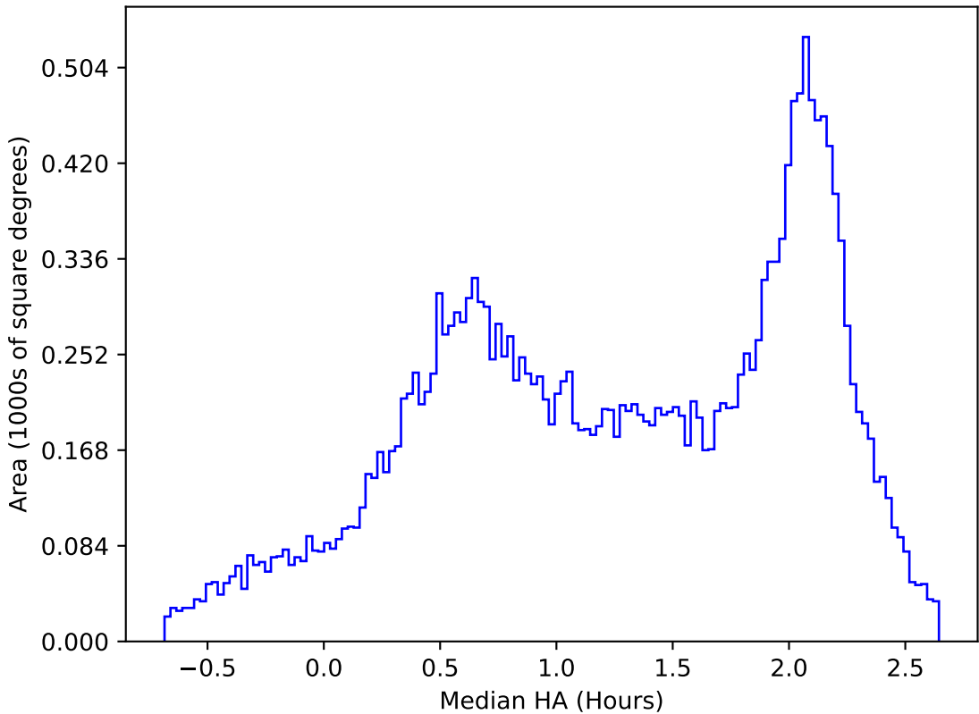
too_elab_r8_d3_ugrizy_v3.4_10yrs All sky y band: Median HA
