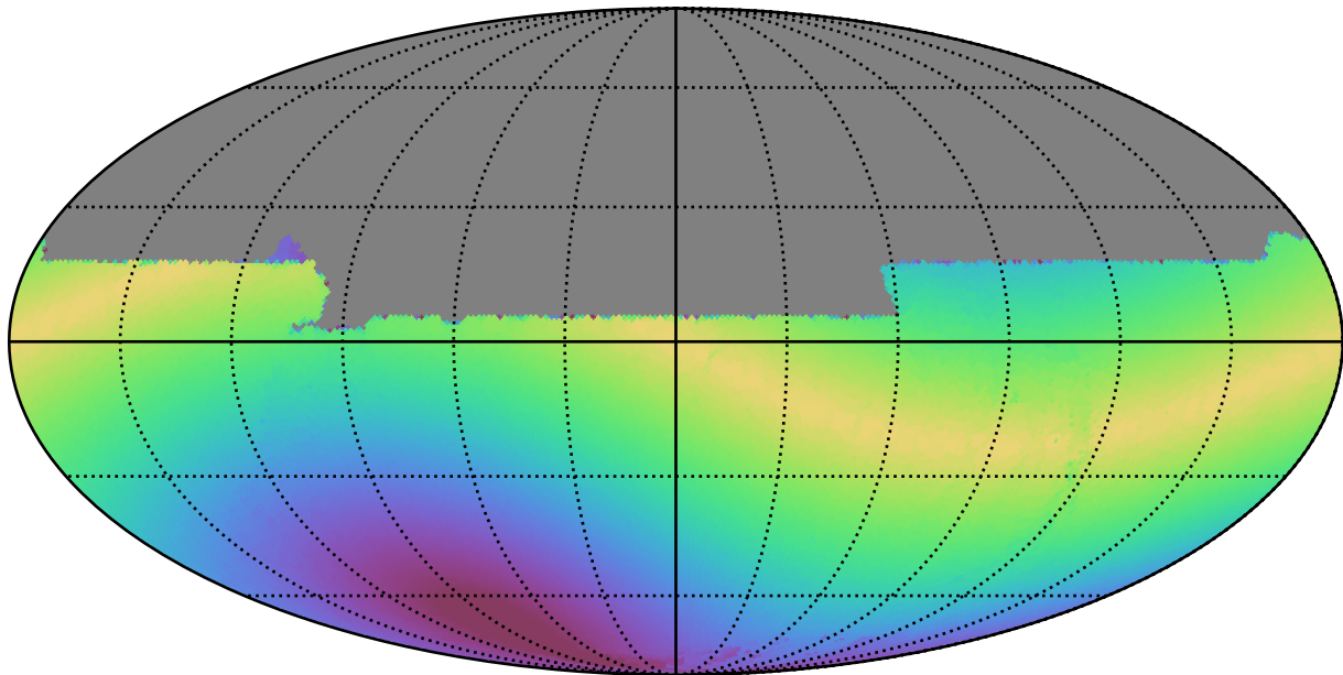
too_elab_r8_d3_ugrizy_v3.4_10yrs All sky y band: Max solarElong
