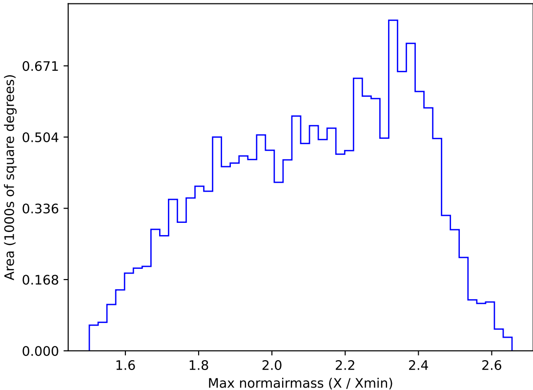
too_elab_r8_d3_ugrizy_v3.4_10yrs WFD r band: Max normairmass
