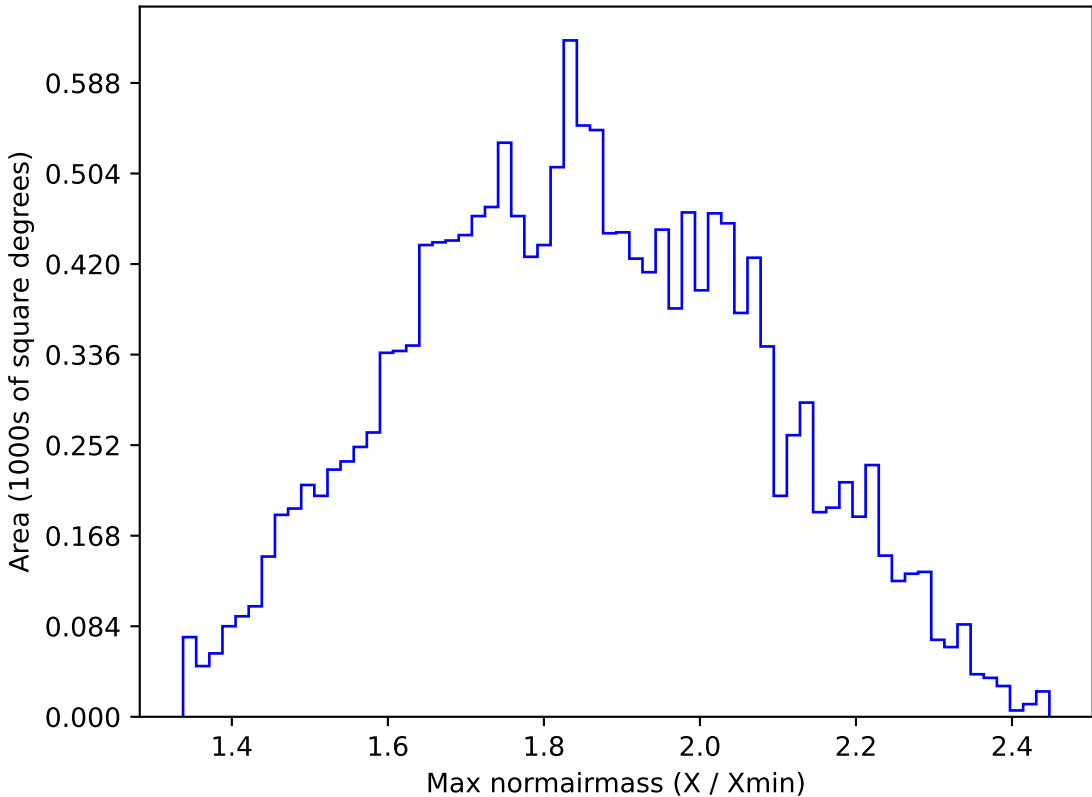
too_elab_r8_d3_ugrizy_v3.4_10yrs WFD g band: Max normairmass
