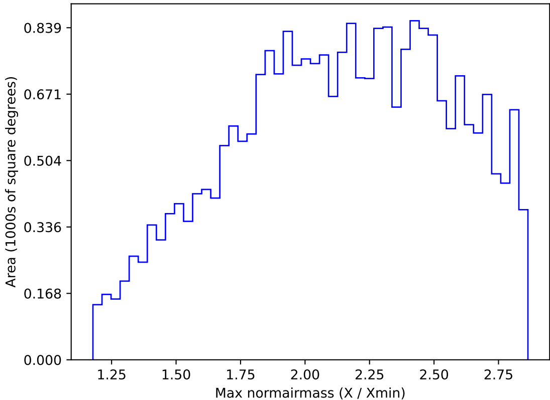
too_elab_r8_d3_ugrizy_v3.4_10yrs All sky z band: Max normairmass
