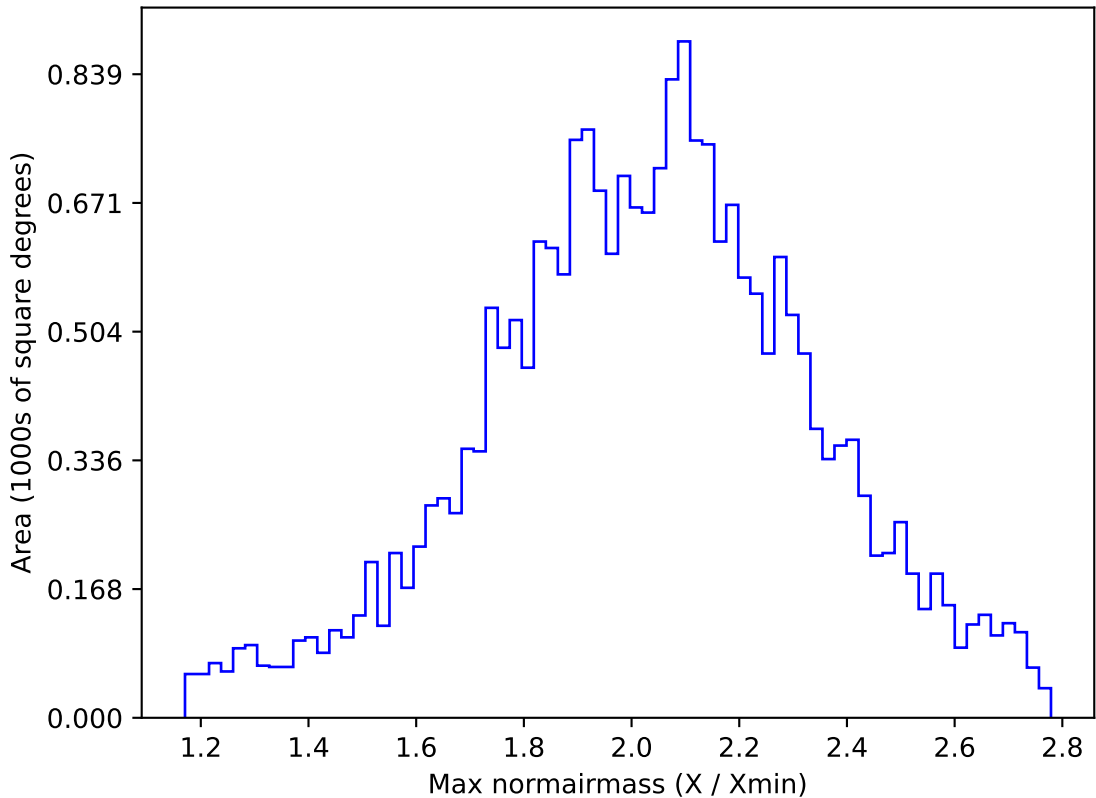
too_elab_r8_d3_ugrizy_v3.4_10yrs All sky y band: Max normairmass
