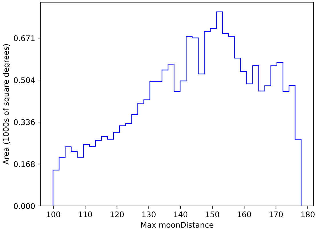
too_elab_r8_d3_ugrizy_v3.4_10yrs WFD y band: Max moonDistance
