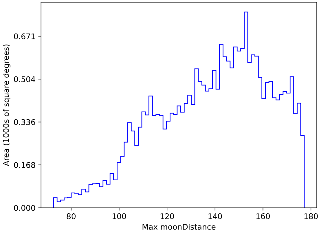
too_elab_r8_d3_ugrizy_v3.4_10yrs All sky y band: Max moonDistance
