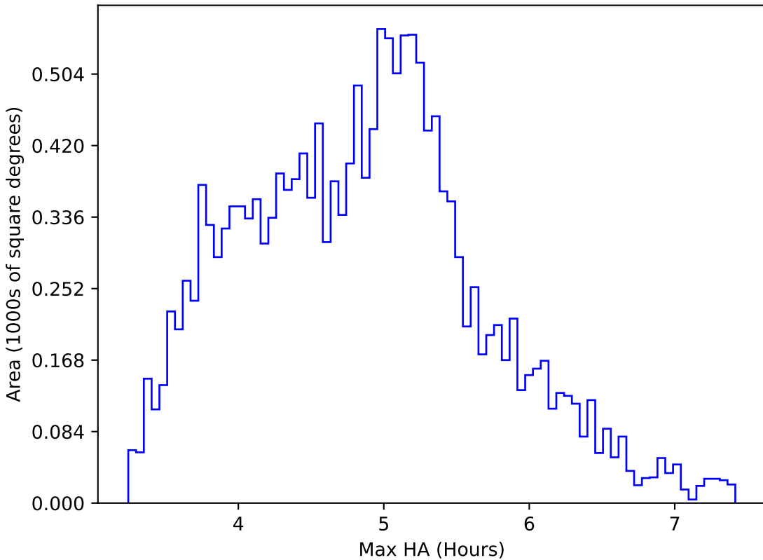
too_elab_r8_d3_ugrizy_v3.4_10yrs WFD z band: Max HA
