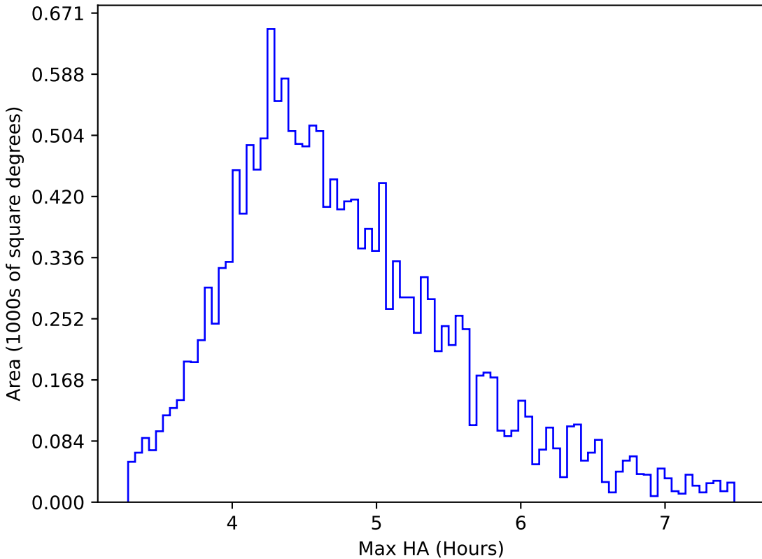
too_elab_r8_d3_ugrizy_v3.4_10yrs WFD y band: Max HA
