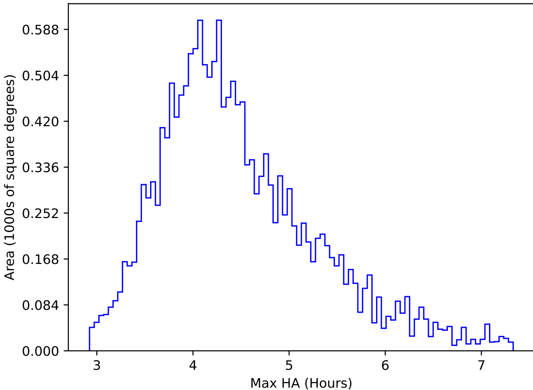
too_elab_r8_d3_ugrizy_v3.4_10yrs WFD r band: Max HA
