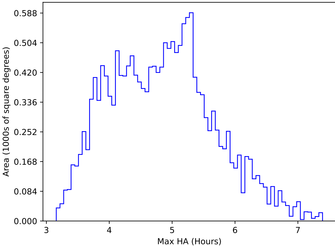
too_elab_r8_d3_ugrizy_v3.4_10yrs WFD i band: Max HA
