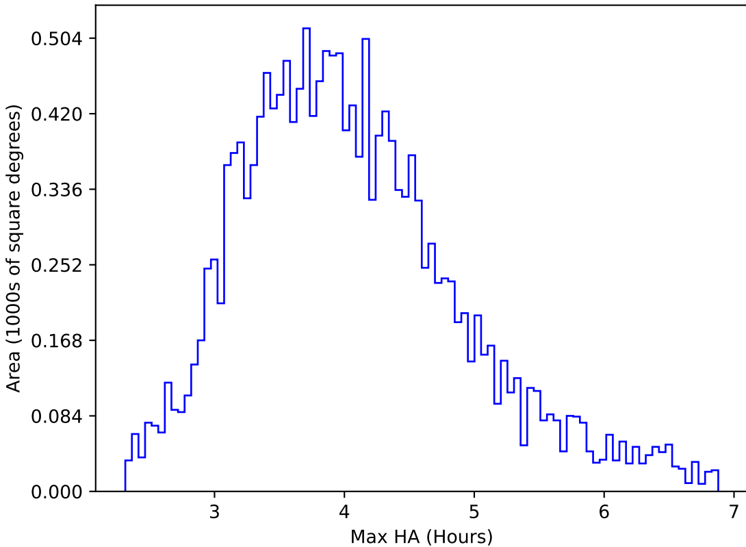
too_elab_r8_d3_ugrizy_v3.4_10yrs WFD g band: Max HA
