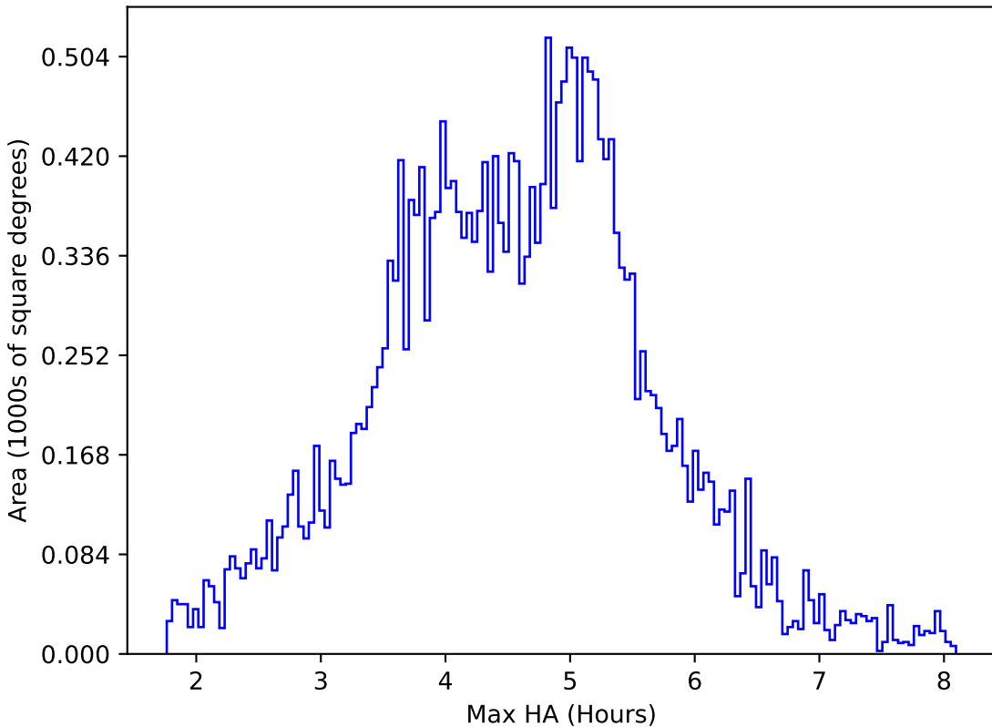
too_elab_r8_d3_ugrizy_v3.4_10yrs All sky z band: Max HA
