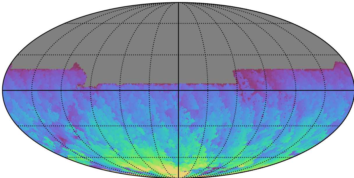
too_elab_r8_d3_ugrizy_v3.4_10yrs All sky y band: Max HA
