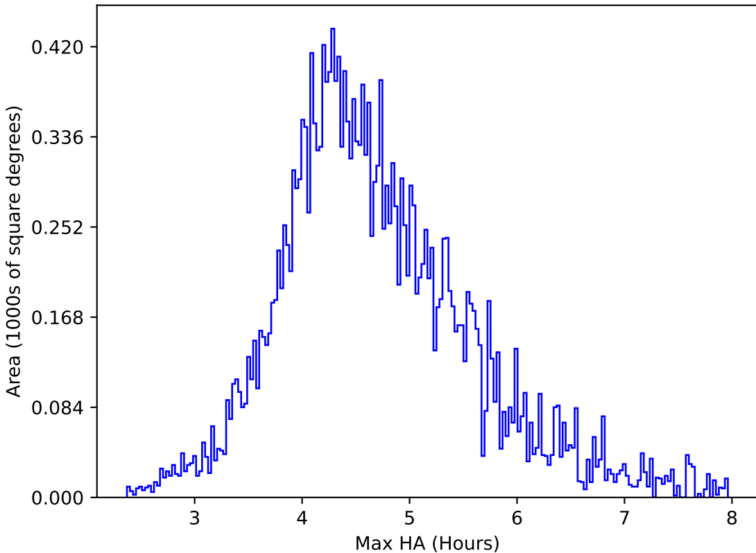
too_elab_r8_d3_ugrizy_v3.4_10yrs All sky y band: Max HA
