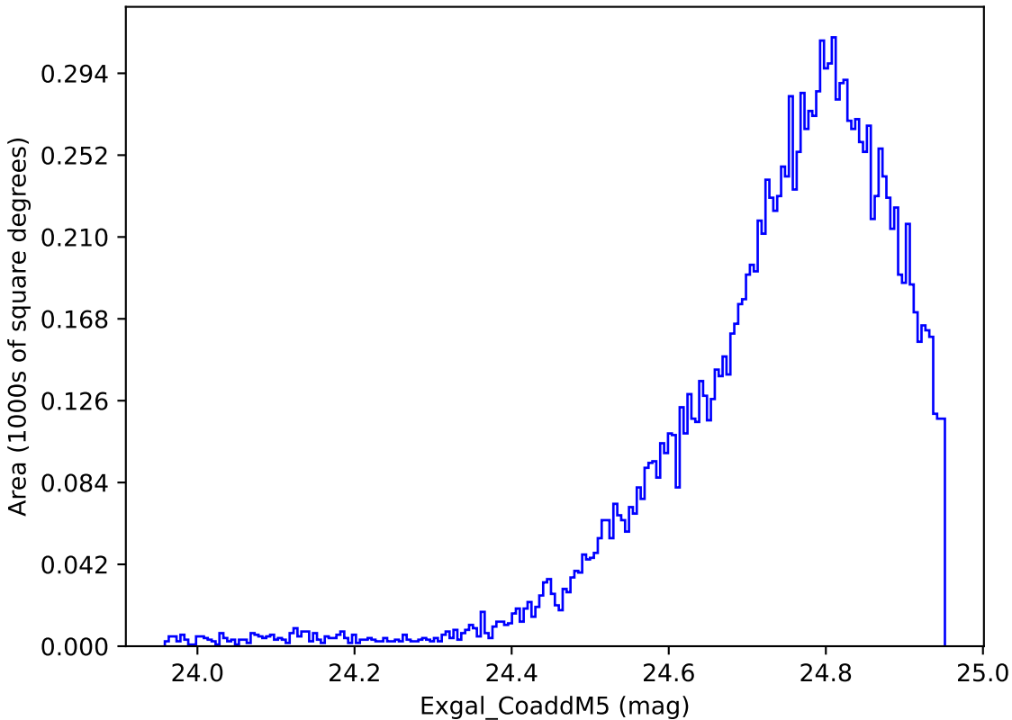
too_elab_r8_d3_ugrizy_v3.4_10yrs WFD y band: Exgal_CoaddM5
