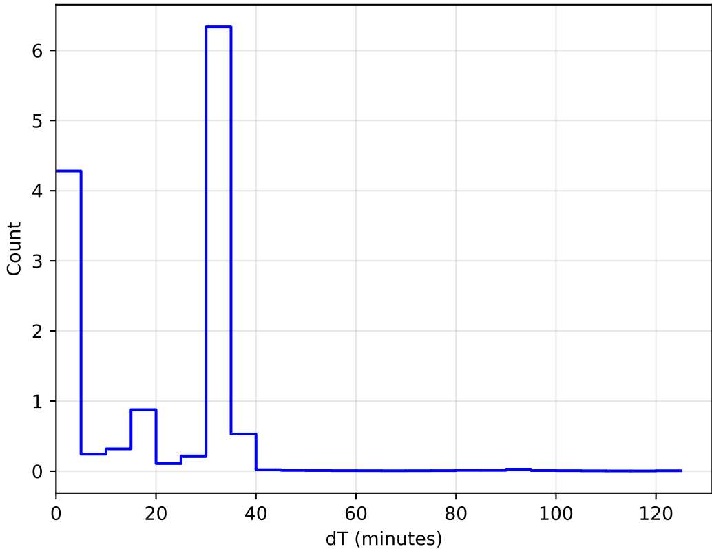
too_elab_r8_d3_ugrizy_v3.4_10yrs All sky: DeltaT Histogram 1e6
