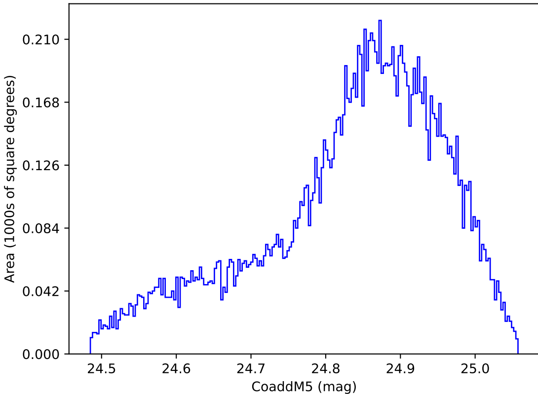
too_elab_r8_d3_ugrizy_v3.4_10yrs WFD y band: CoaddM5
