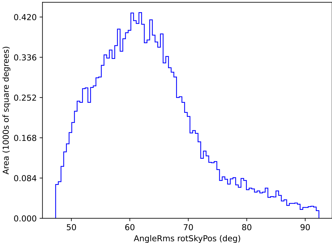
too_elab_r8_d3_ugrizy_v3.4_10yrs WFD y band: AngleRms rotSkyPos
