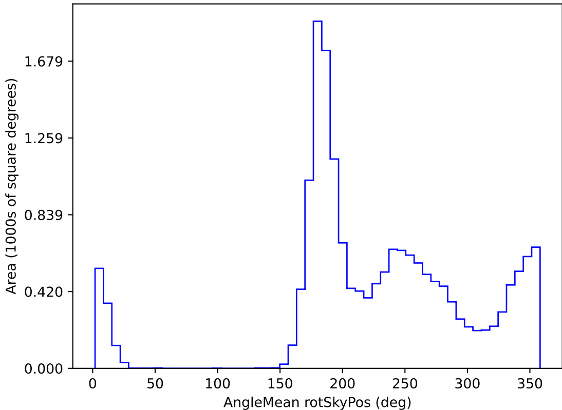
too_elab_r8_d3_ugrizy_v3.4_10yrs WFD y band: AngleMean rotSkyPos
